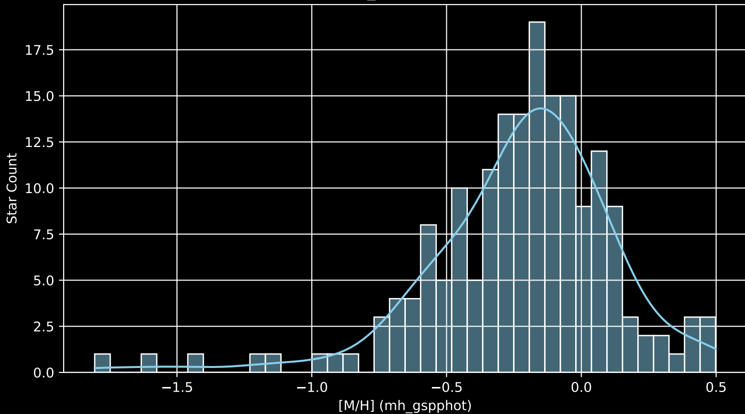
APOGEE DR17 Field: [053+40 MGA [M/H] (mh_gspphot) (n= 179)
